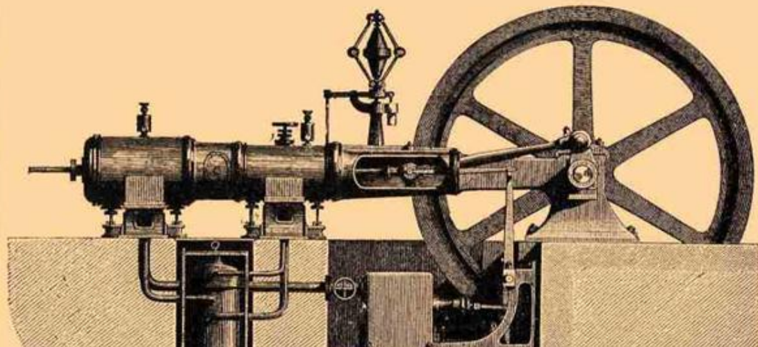
1. Горизонтальная паровая машина съ парораспределителем Зульцера
